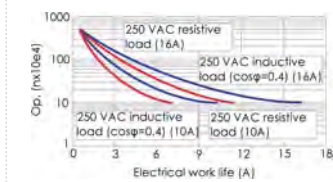
Vida eléctrica RFS2-PT
