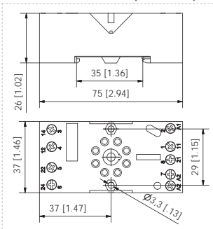
Dimensiones SM2 (mm-inch)
