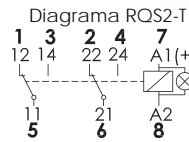
RQS1-T Relé 1 contacto RQS2-T Relé 2 contactos RQS4-T Relé 4 contactos
