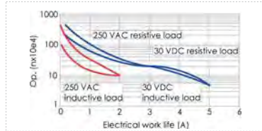
Vida eléctrica RQS4-T
