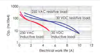
Vida eléctrica RQS1-RQS2
