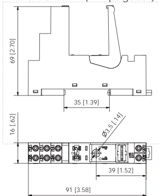
Dimensiones SF2 (mm-pulgadas)
