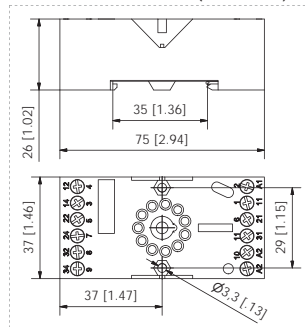
Dimensiones SM3 (mm-inch)
