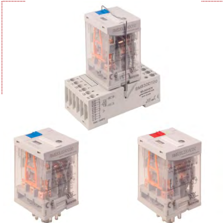
RMS2 Relé 8 pines 2 contactos
